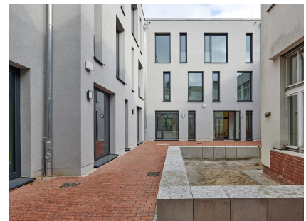
Die Erweiterungsbauten schließen direkt an das vielgliedrige Gebäude an. Daraus ergibt sich ein weiterer geschlossener Innenhof
