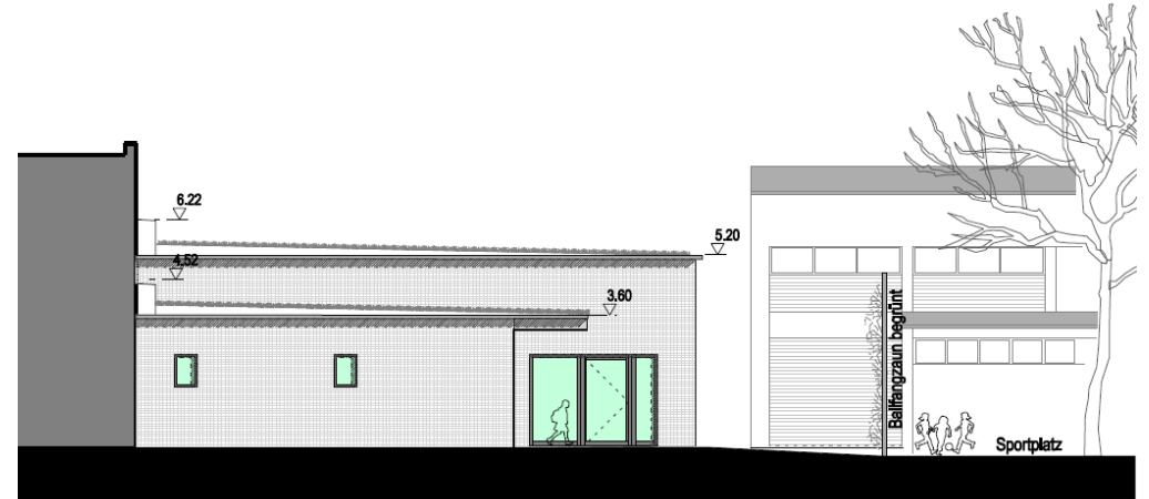
Ansicht Nord
