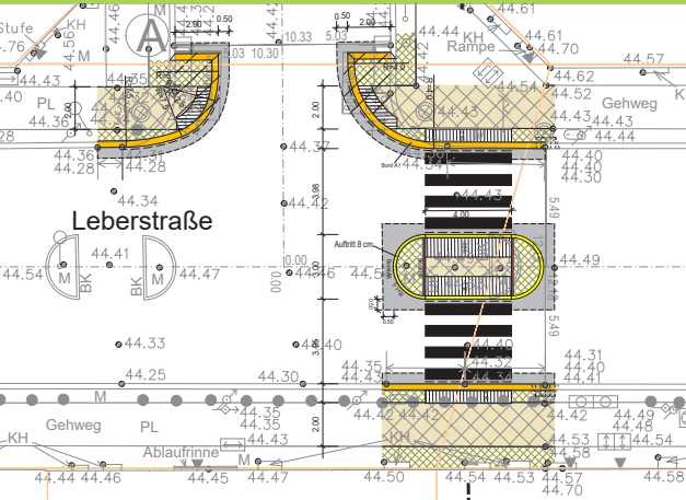
Planung für die barrierefreie Querungsstelle Leberstraße
