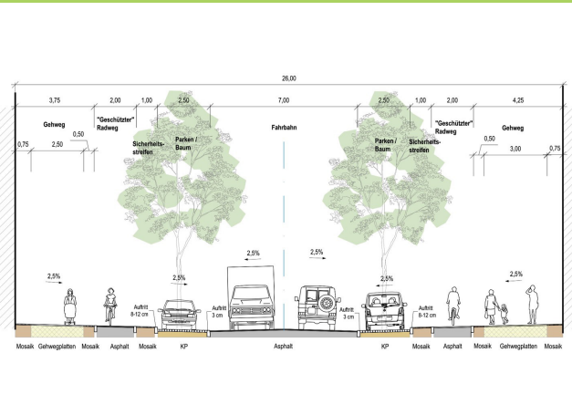
Straßenquerschnitt für den Tempelhofer Weg
