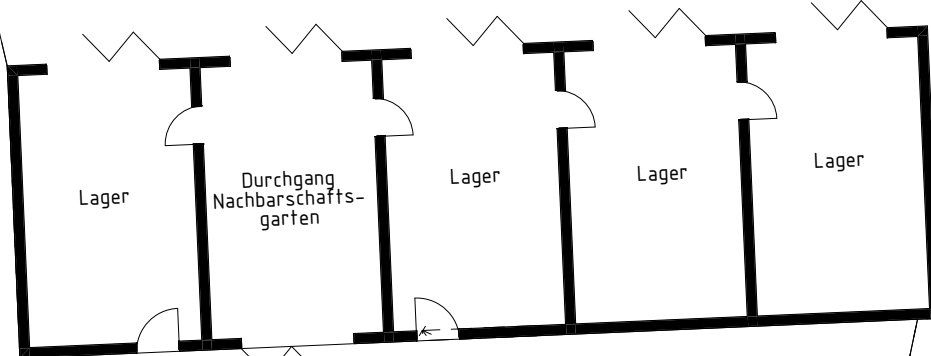
Grundriss Erdgeschoss
